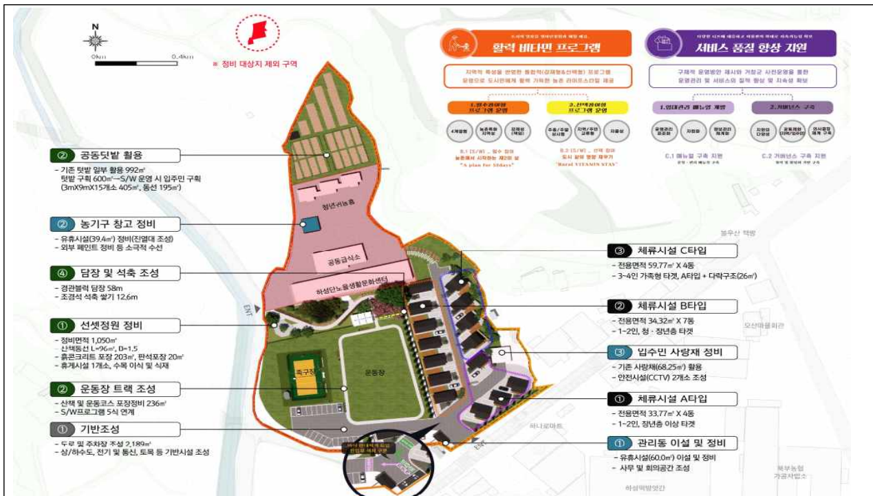
기본계획 종합계획도
