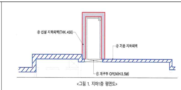
장비 반입구(3m*5m) 평면도
