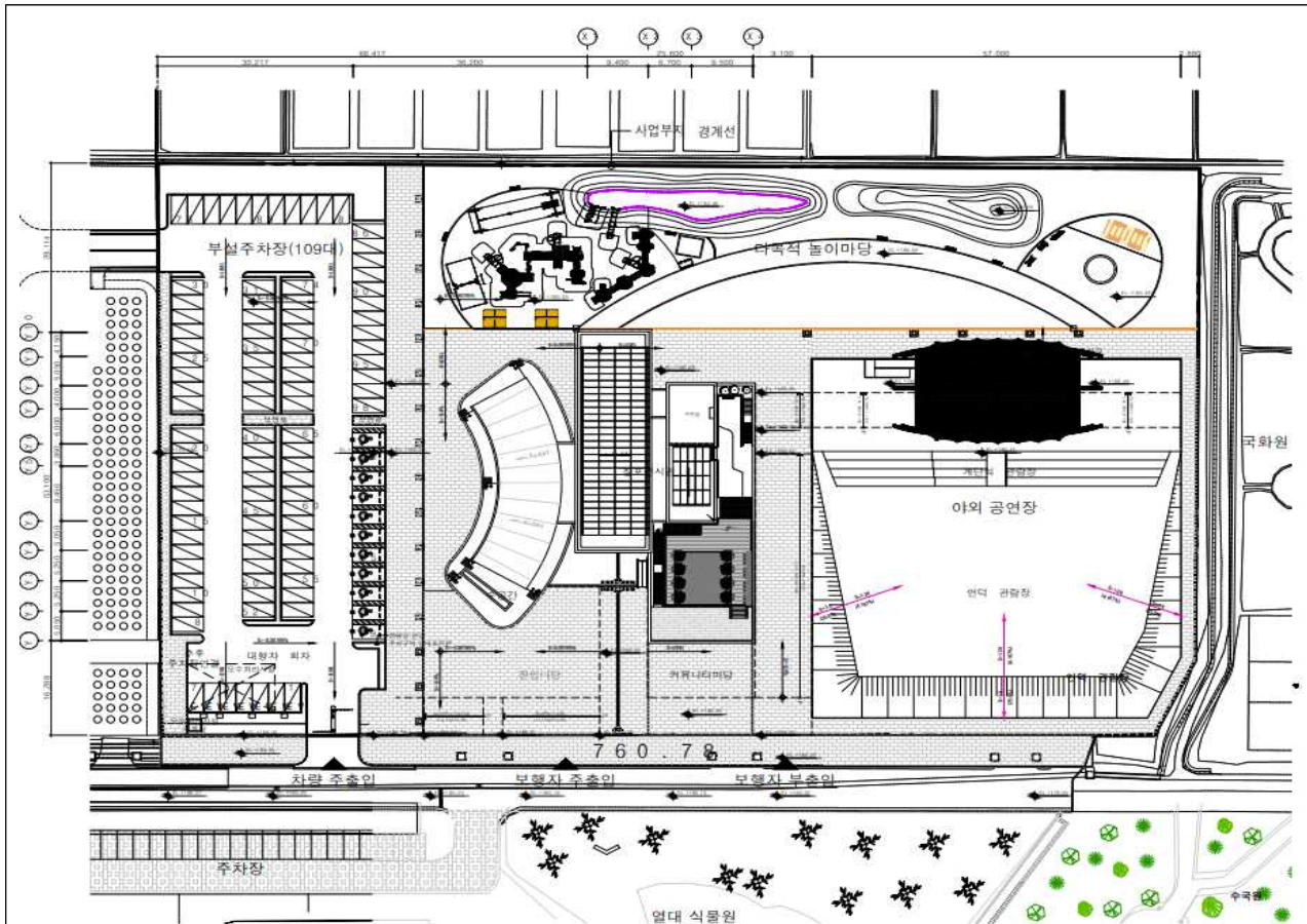
배치도
